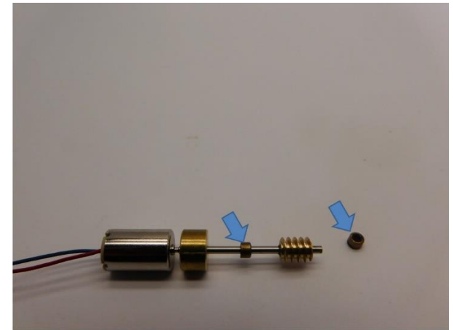
Die Metallteile sind verklebt (Lager nicht kleben) The metal parts are glued (Don't glue the bearings) De metaaldelen zijn verlijmd (Verlijm de lagers niet)
