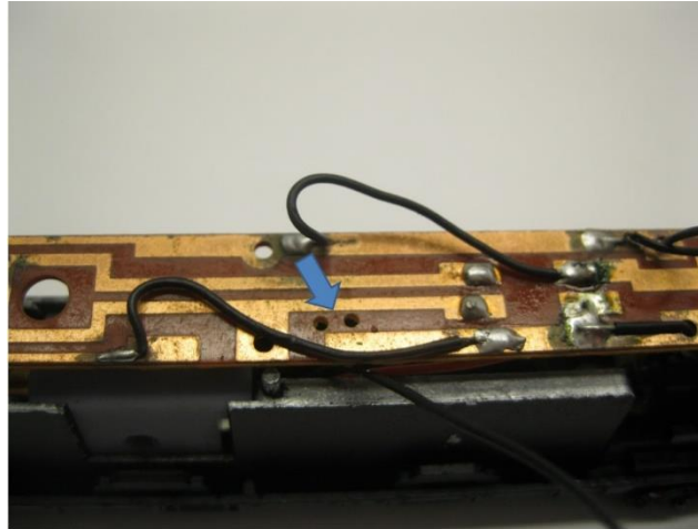
Bohren Sie 2 kleine Löcher Drill 2 small holes Boor 2 kleine gaten
