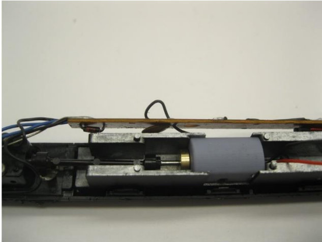
Platzieren Sie die Motor mit ein Kardankupplung Mount the motor with one cardan coupling Plaats de motor met een kardan koppeling
