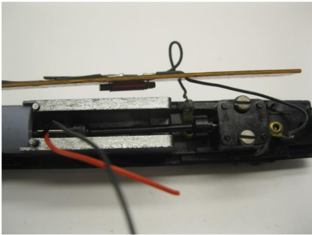
Kardanwelle platzieren Mount the cardan shaft Plaats de kardan as
