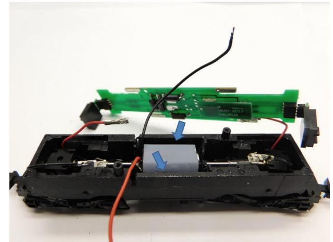
Kleben Sie den Motor Glue the motor Lijm de motor
