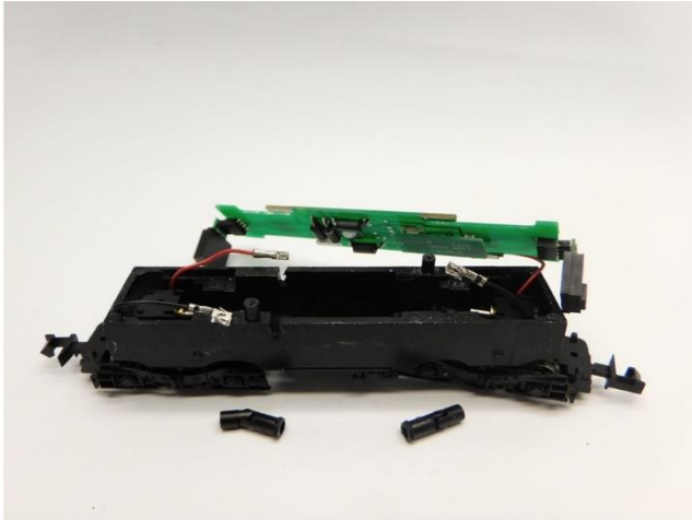
Kardankupplungen entfernen Remove cardan couplers Verwijder de kardankoppelingen
