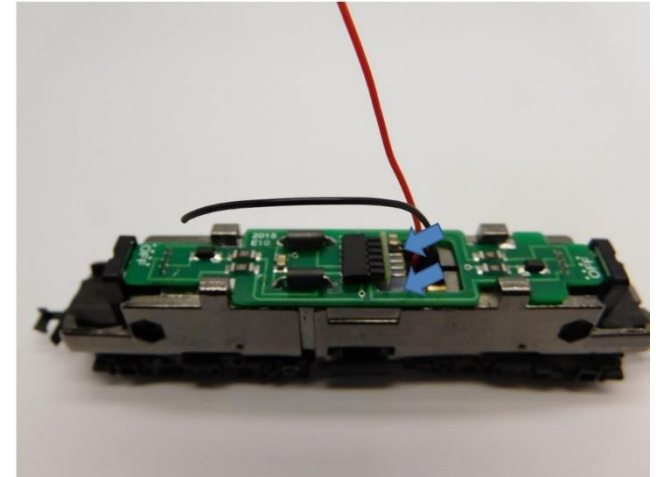
Motor am Gehäuse kleben Glue motor to the frame Verlijm de motor tegen het frame
