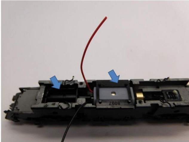
Deckel platzieren Mount the covers Plaats de afdekkingen
