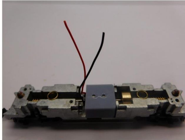
Lager platzieren Mount the bearings Plaats de lagers
