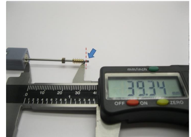
Die Achse muss noch gekürzt werden The axle still needs to be shortened De as moet ingekort worden
