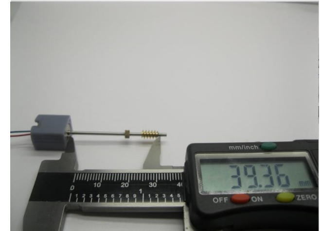
Klebe die Schnecke Glue worm gear Verlijm het wormwiel
