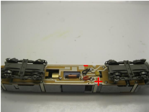
Drehgestellen platzieren und löten Sie die Drähte Mount bogies and solder the wires Plaats de draaistellen en soldeer de draden
