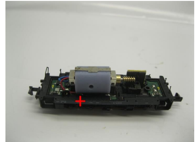
Löten Sie die Drähte und Klemme plätzen Solder the wires and mount motor clamp Soldeer de draden
