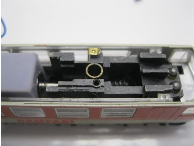
Messingbuchs platzieren Mount brass bushing Plaats het messing lager
