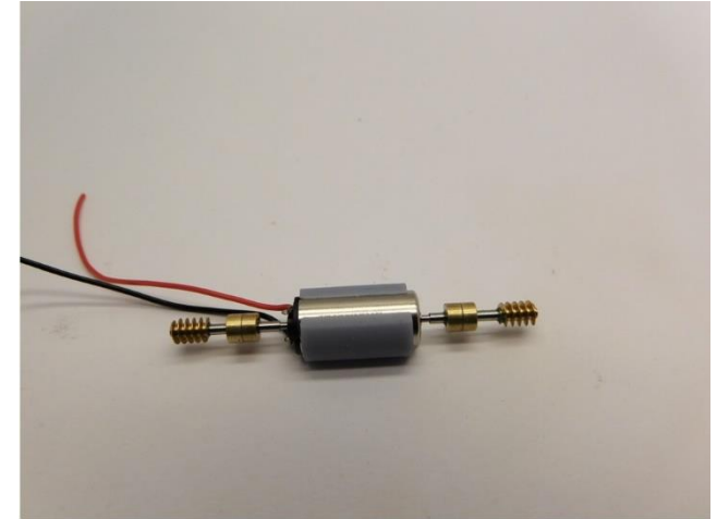
Der Motor wird mit Epoxidkleber oder Sekundenkleber zwischen den Motorhalter eingeklebt The motor is glued between the motor holder with epoxy glue or super glue De motor wordt verlijmd tussen de motorhouder met secondelijm of epoxy lijm
