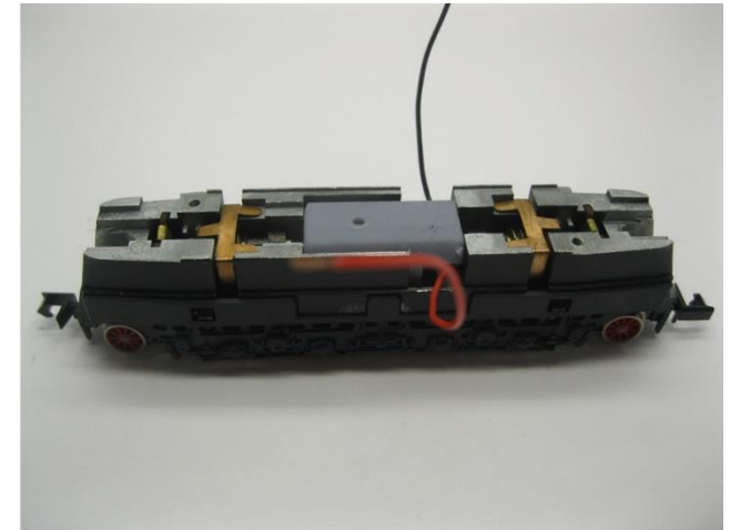
Drehgestellseiten platzieren Mount bogie sides Plaats draistel zijkanten
