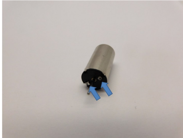
Biegen Sie die Lötlippen Bend the soldering lips Buig de contacten
