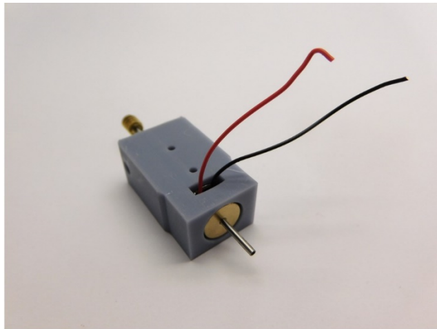
Platzieren Sie die 2e Schwungmasse und Schnecke Mount the 2nd flywheel and worm gear Plaats het 2e vliegwiel en wormwiel
