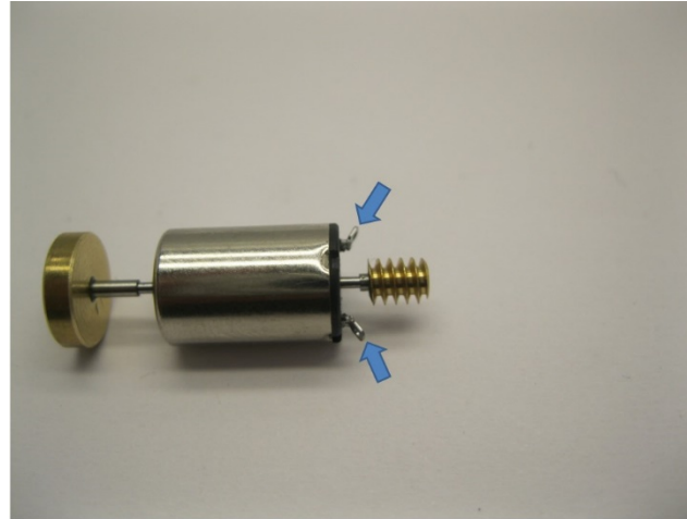
Biegen Sie die Kontakte wie im Bild gezeigt Bend the contacts as shown in the picture Buig de contacten zoals in de afbeelding
