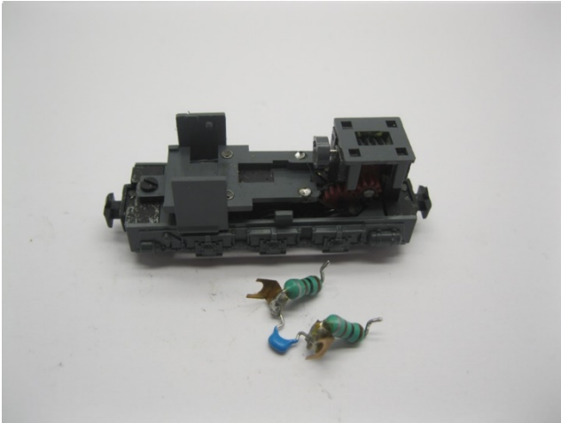
Entfernen Sie die Entstörteile Remove the interference suppression parts Verwijder de ontstoordeelen
