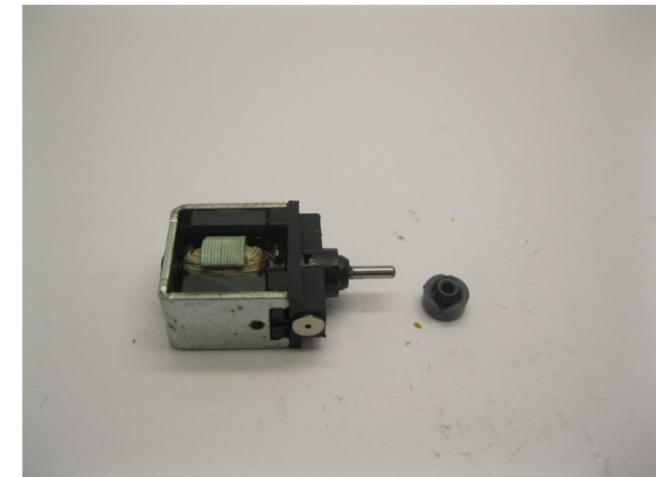
Sie brauchen dieses Teil wieder. Diese wird mit einer Pinzette entfernt You need the part again. It can be removed with tweezers Je hebt dit onderdeel wederom nodig. Het kan met een pincet verwijderd worden
