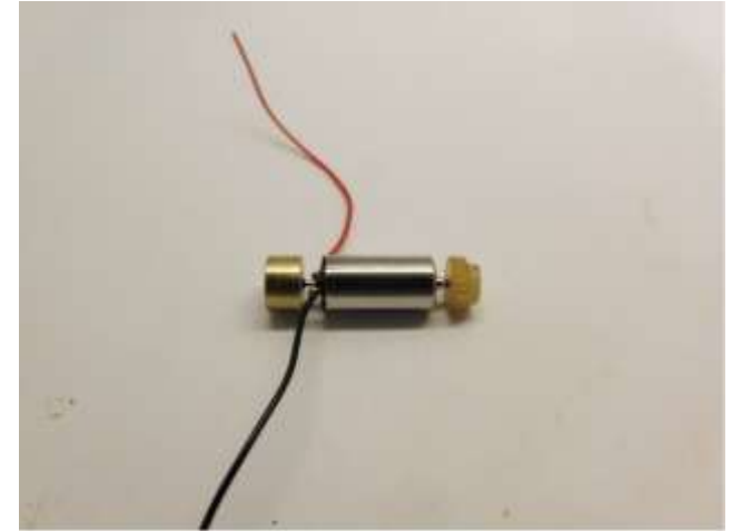
Wellen mit ein Trennscheibe kürzen Shorten the shafts with a cutting disc Kort de assen in met een slijpschijf
