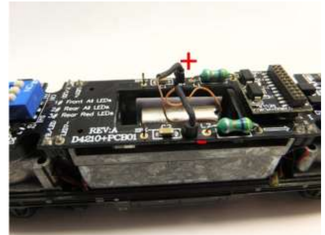
Verbinde die Drähte Connecting wires Sluit de draden aan
