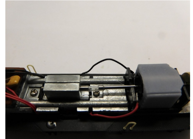
Schlauchkupplung kleben Glue the hose coupling Verlijm de slangkoppeling
