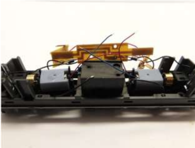
Platzieren Sie den Motoren Place the motors Plaats de motoren
