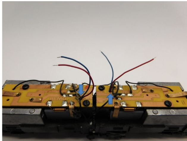
Bohren Sie 2 Löcher für die Drähte Drill 2 holes for the wires Boor 2 gaatjes voor de draden
