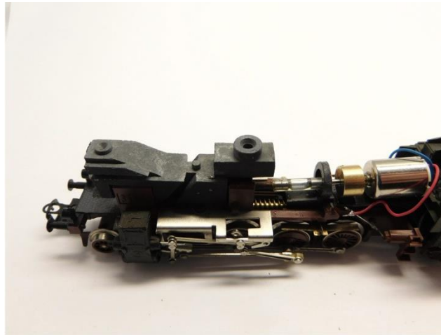
Gewicht platzieren Mount weight
