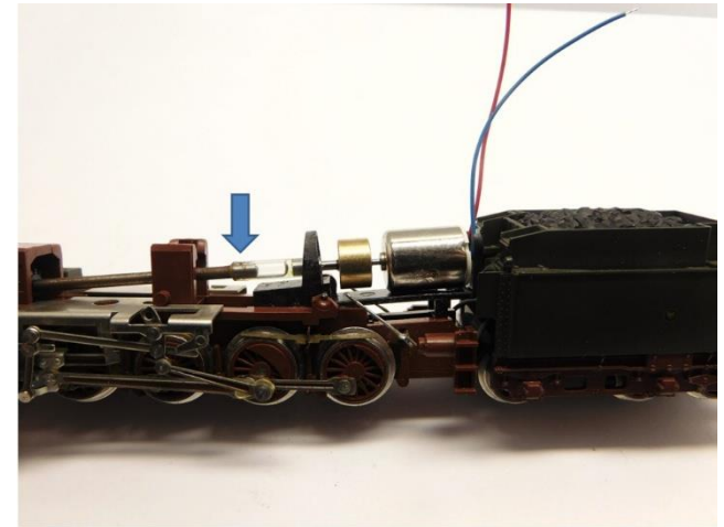
Schlauchkupplung kleben Glue the hose coupling
