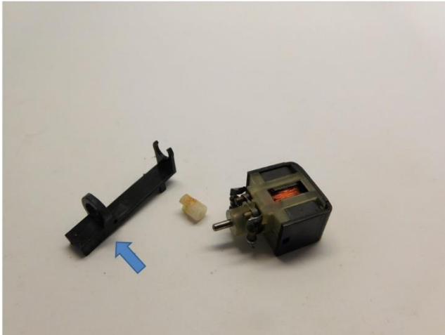
Sie brauchen dieses Teil wieder You need the part again
