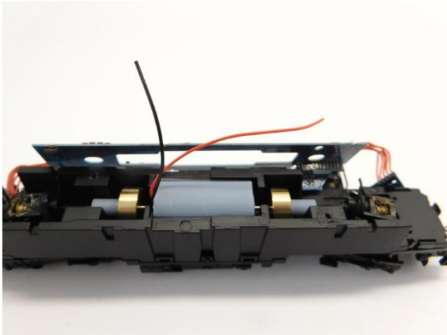
Motor plaatsen Place the motor Plaats de motor
