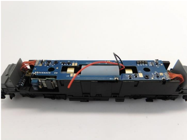
Platine plaatsen Place the PCB Plaats de printplaat
