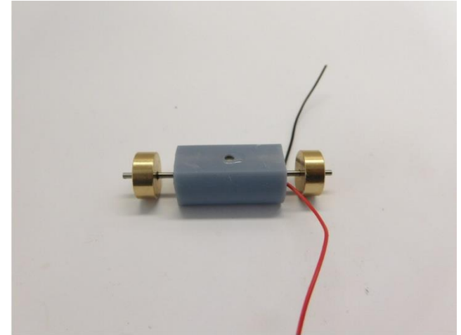
2e Schwungmasse kleben Glue 2nd flywheel Verlijm het 2e vliegwiel
