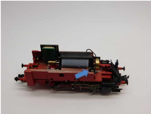
Roco Motorhalter platzieren Mount the Roco motor mount Plaats de Roco motor houder
