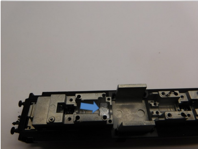
Schwungmasseraum vergrößern Increase flywheel space Vergroot de ruimte voor het vliegwiel
