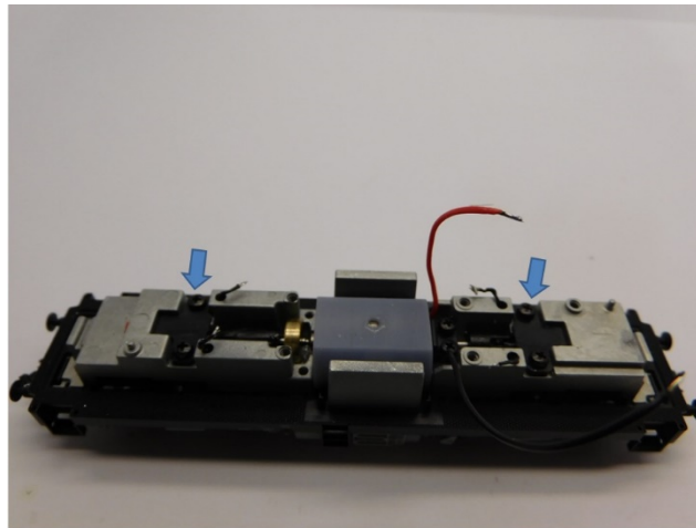
Schnecken-Abdeckbleche montieren Mount worm gear cover plates Plaats de wormwiel afdekplaten
