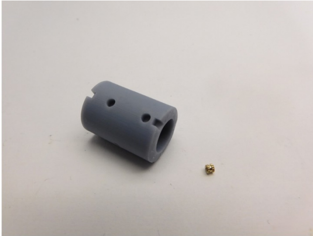
Die Messingeinsatz wird mit Sekundenkleber in den Motorhalter eingeklebt The brass inserts is glued into the motor holder with superglue De messing insert wordt met secondelijm verlijmd in de motor houder
