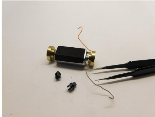
Sie brauchen diese Teile wieder. Diese werden mit einer Pinzette entfernt You need the parts again. They can be removed with tweezers
