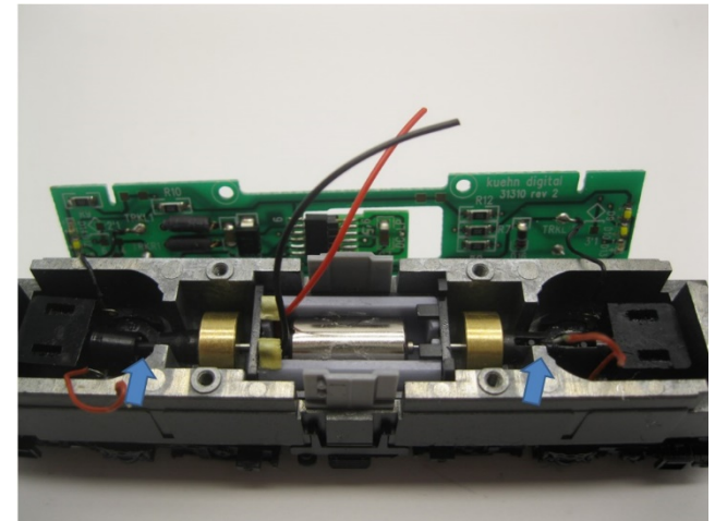
Kardangelnkupplungen platzieren Mount cardan couplings Plaats de cardankoppelingen
