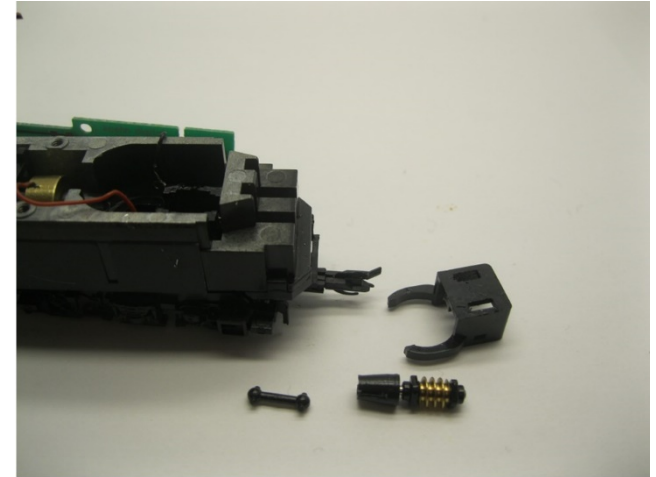
Getriebedeckel abnehmen Remove gear cover Verwijder het wormwieldeksel
