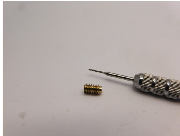
Prüfen Sie ob das Loch 1 mm groß ist Check that the hole is 1mm Controleer of het gat 1 mm is
