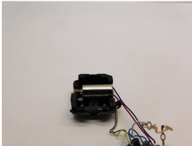
Prüfen Sie, ob der Motor passt Check whether the motor fits Controleer of de motor past
