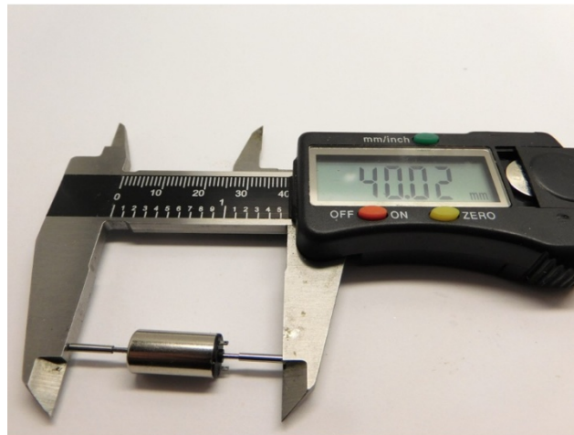
Maße prüfen (10 mm Wellen) Check dimensions (10 mm shafts) Controleer de maatvoering
