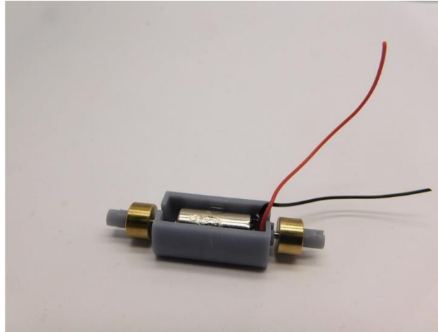
Kardankupplungshalter platzieren Mount the cardan coupler holders Monteer de kardankoppelingshouders
