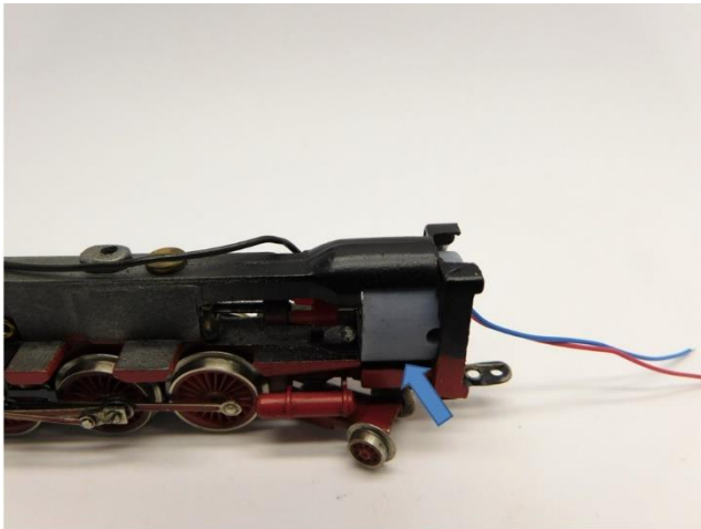
Motor kleben Glue motor Verlijm motor
