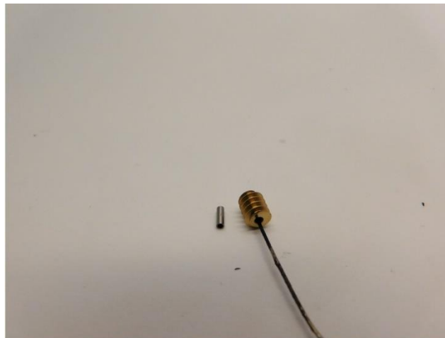
Tragen Sie Klebstoff auf die Innenseite von die Teile Apply glue on the inside of the parts Plaats alleen lijm aan de binnenzijde van de onderdelen
