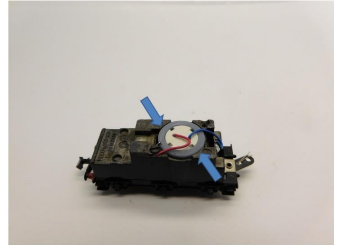
Motor kleben Glue motor Vijrlijm de motor
