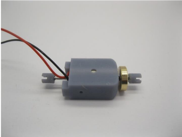
Kleben Sie die kurze Kardankupplungshalter mit Sekundenkleber Glue the short cardan couplerholders with superglue Verlijm de kardankoppelingshouders met secondelijm
