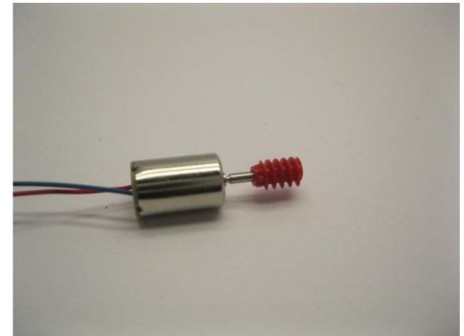
Kleben Sie die Schnecke mit einem Tropfen Sekundenkleber auf den Welle Glue the worm on the shaft with a drop of superglue Lijm het wormwiel met een druppel secondelijm
