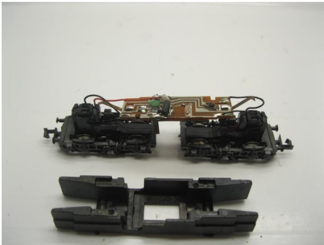
Drehgestelle ausklipsen Unclip bogies Draaistellen losklikken
