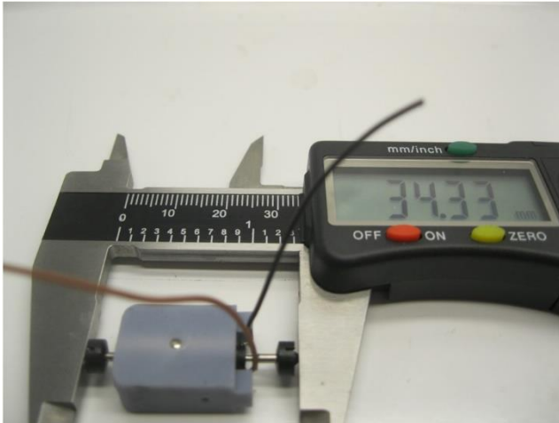
Federnaben kleben und prüfen Glue and check spring caps Verlijm de veerkoppelingen en controleer de maten
