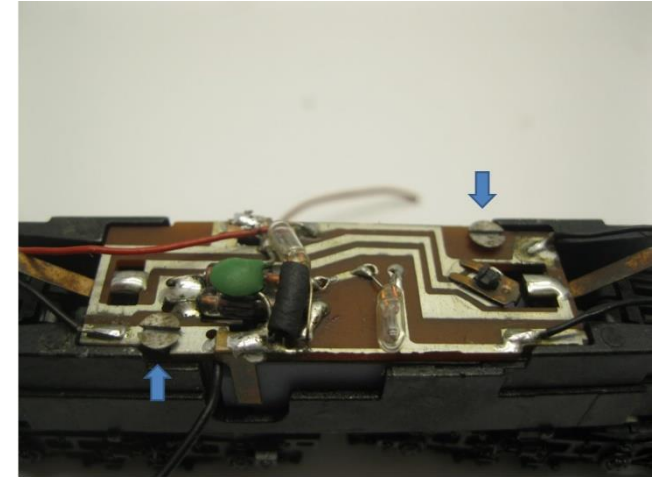
Platine plätzen Mount the PCB Plaats de printplaat
