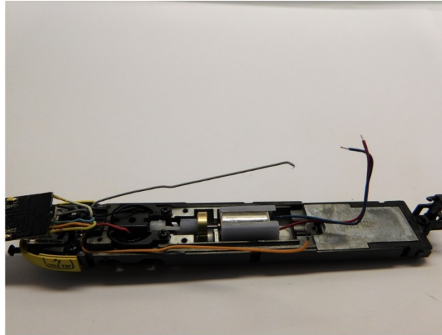
Erste Motor platzieren Mount the first motor Plaats de eerste motor
