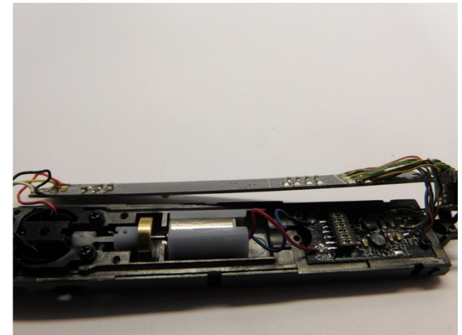
Zweite Motor platzieren Mount the second motor Plaats de tweede motor
