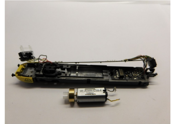
Ausbau zweiter Motor Take out the second motor Demonteer de tweede motor
