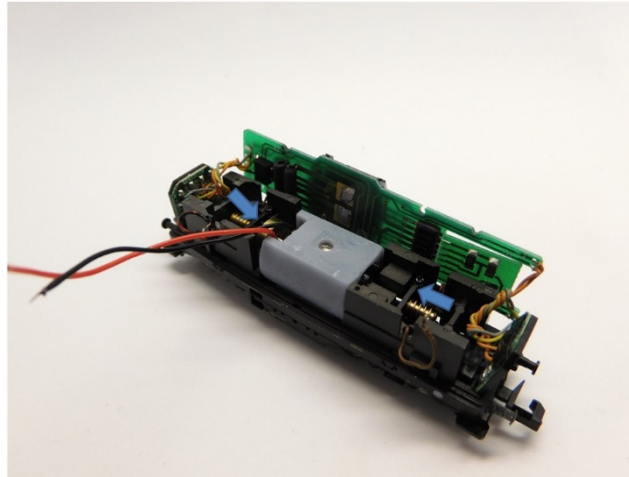
Platzieren Sie den Klemmen Mount the motor clamps Plaats de motorklemmen
