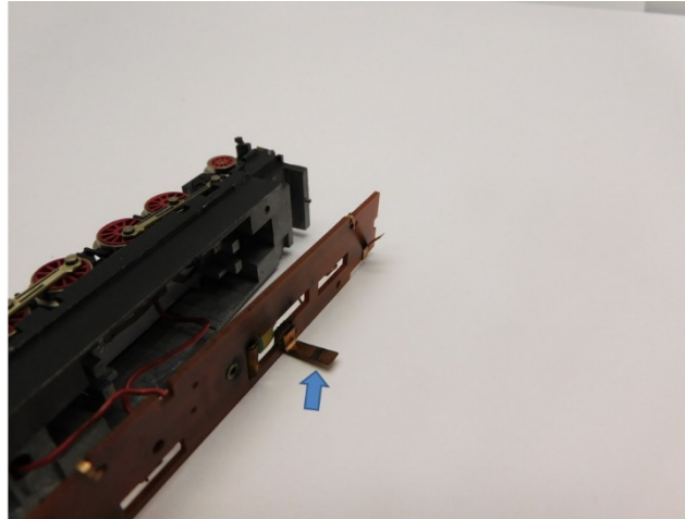
Alter Motorkontakt entfernen Remove old motor contact Verwijder het oude motorcontact
