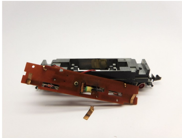
Alter Motorkontakt entfernen Remove old motor contact Verwijder het oude motorcontact
