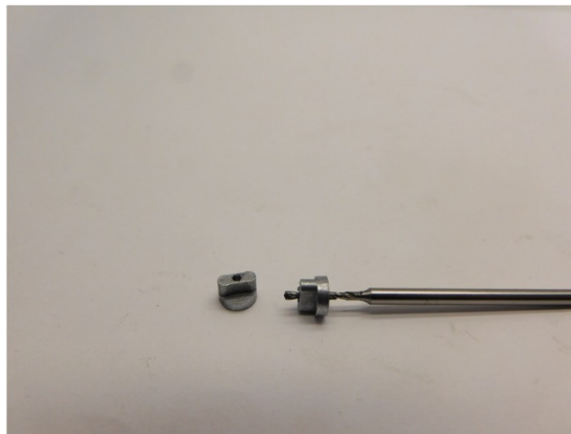
Loch auf 1.5 mm vergrößern Enlarge the hole to 1.5 mm Vergroot het gat naar 1.5 mm
