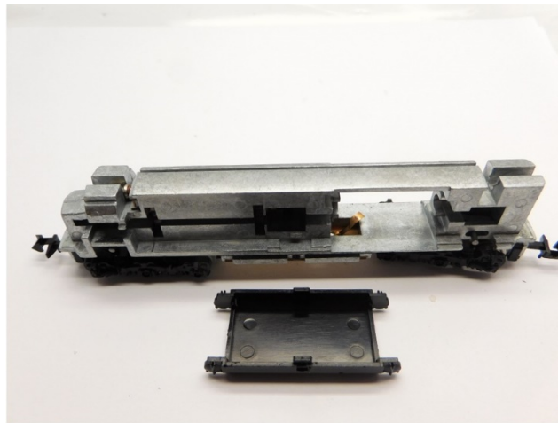
Bodenplatte abnehmen Take off bottom plate Bodemplaat afnemen
