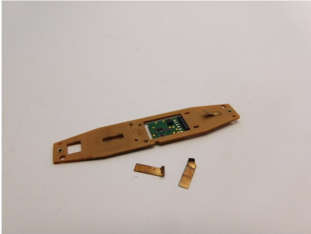
Alter Motorkontakten entfernen Remove old motor contacts Verwijder de oude motorcontacten
