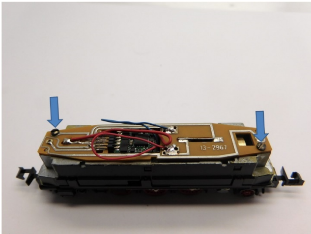
Leiterplatte platzieren Mount circuit board Plaats de printplaat
