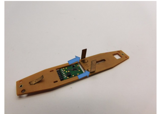
Alter Motorkontakten entfernen Remove old motor contacts Verwijder de oude motorcontacten
