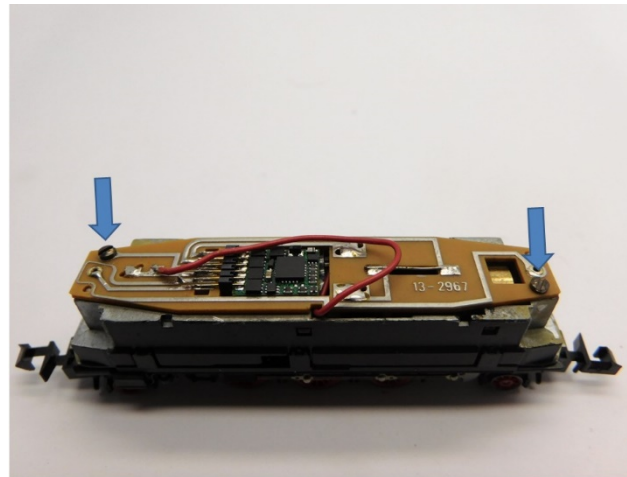
Entfernen sie die Leiterplatte Remove the circuit board Demonteer de printplaat
