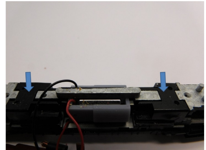
Gewichte platzieren Mount weights Gewichten plaatsen
