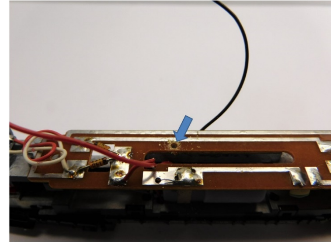
Bohren Sie ein Loch in die Leiterplatte Drill a hole in the PCB Boor een gat in de printplaat
