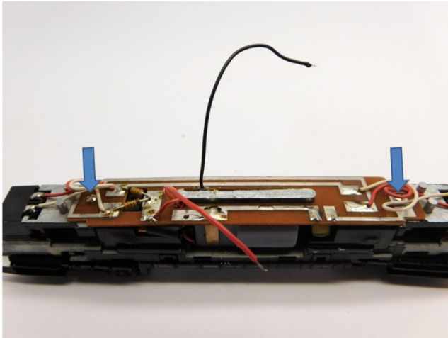
Leiterplatte platzieren Mount PCB Plaats printplaat
