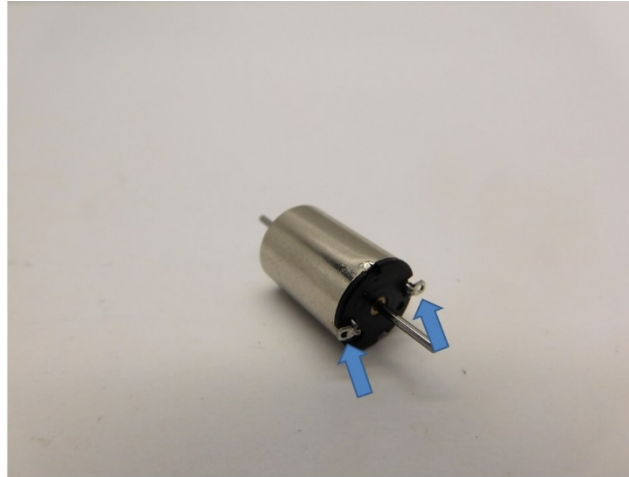
Biegen und kürzen Sie die Lötlippen! Bend and shorten the soldering lips! Buig de contacten en kort ze in!
