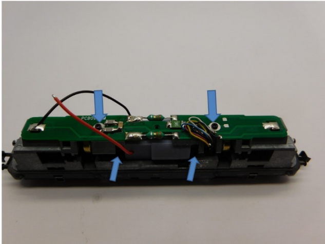
Leiterplatte und Klemmen platzieren Mount circuit board and clamps Plaats de printplaat en de klemmen
