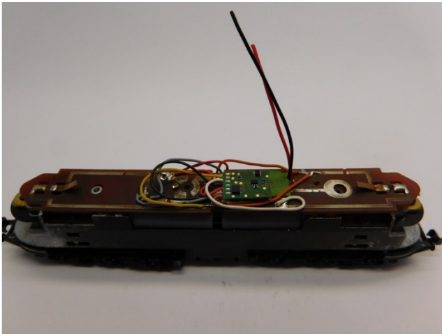
In diesem Fall wird die Verkabelung an den Decoder angeschlossen In this case the wiring is connected to the decoder In dit geval wordt de draden aan een decoder aangesloten
