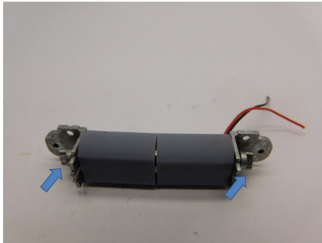
Kardankupplungen platzieren Mount cardan couplers Plaats de cardan koppelingen
