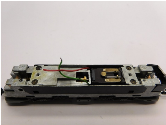
Bei Minitrix 51 1004 00 (mit 2 Motoren) müssen 2 Umbausätze NM038G gekauft werden. With Minitrix 51 1004 00 (with 2 motors) 2 upgrade kits NM038G must be purchased.
