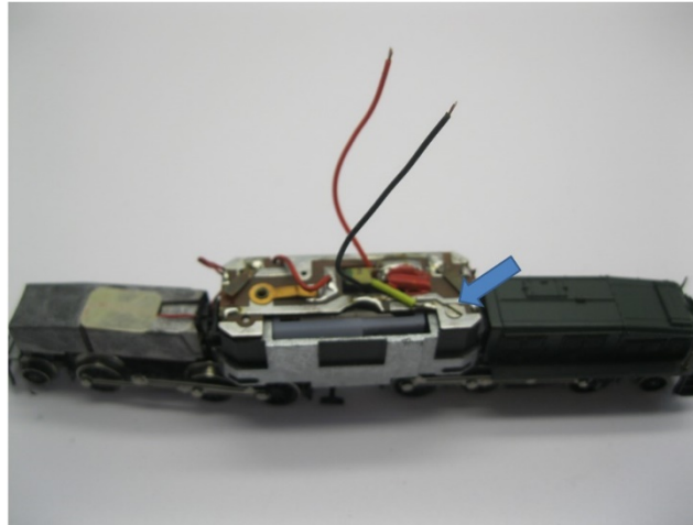
Platine plaziieren Mount PCB Plaats de printplaat
