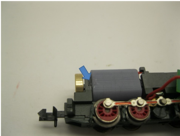
Der Motor wird mit Epoxidkleber oder Sekundenkleber an den Gehäuse geklebt The motor is glued to the frame with epoxy glue or super glue De motor wordt aan het frame verlijmd met secondelijm of epoxy lijm
