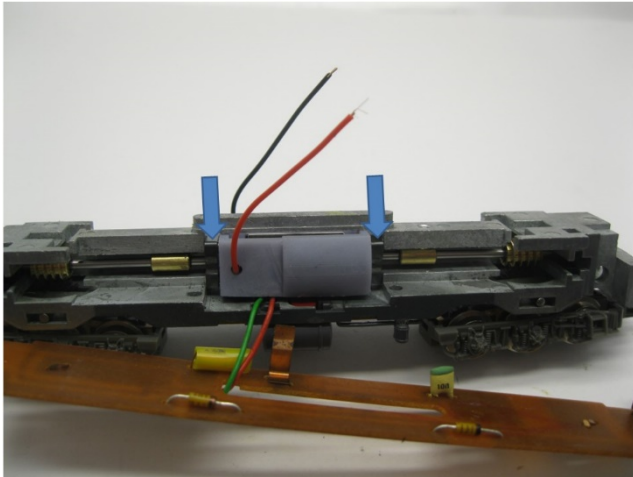
Klemmen platzieren Mount clamps Plaats de eklemmen
